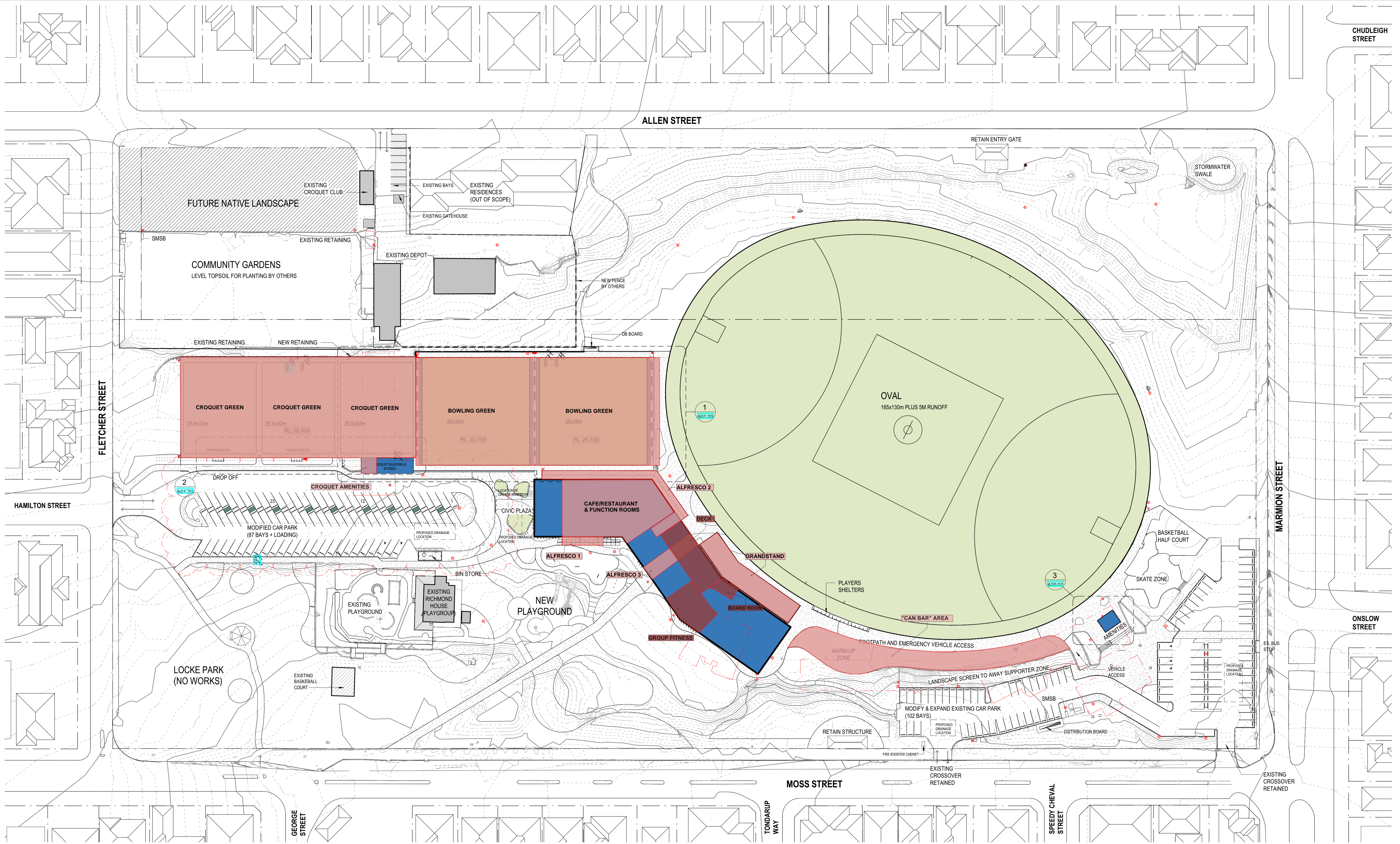
SITE PLAN 1:600
